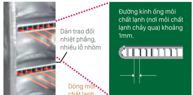
Dàn trao đổi nhiệt Microchannel
