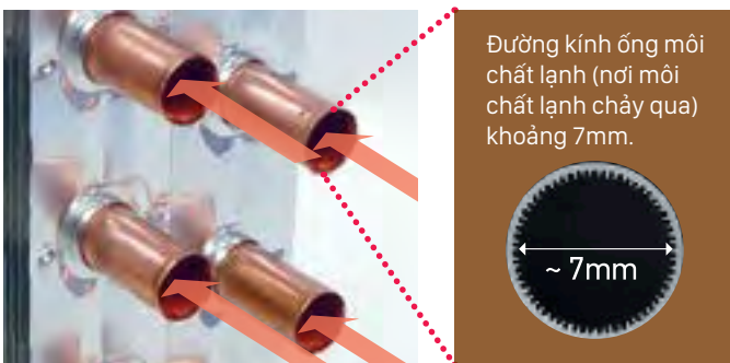
Ống và cánh tản nhiệt thông thường
